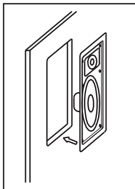
4) Verdrahtung am Lautsprecher festmachen
